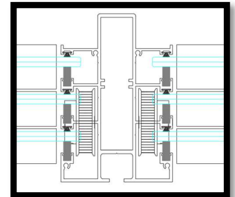
DET. T-3000N 2/3 A. INVERSA
