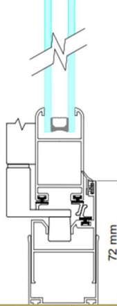
GUÍA SUPERPUESTA
