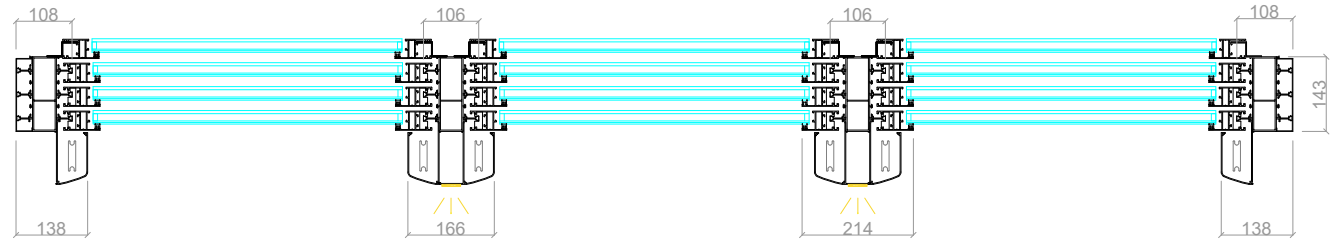
Sección Frontal
