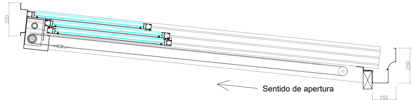
Sección Lateral - Abierto
