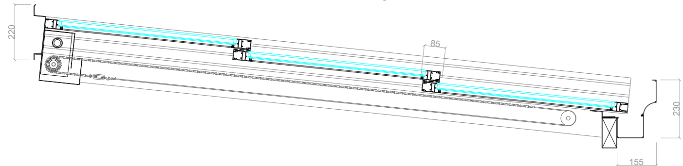
Sección Lateral - Cerrado
